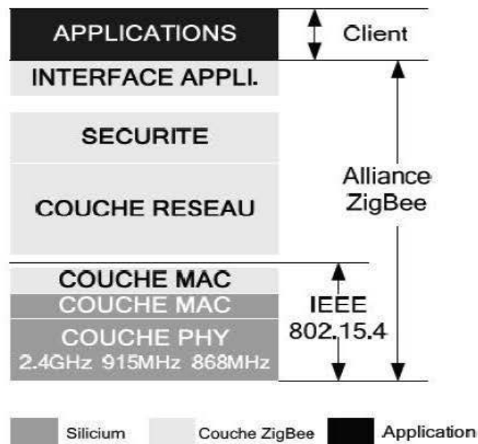
Figure 2. 7: Différence entre l’alliance ZigBee et le standard IEEE 802.15.4 [2]
