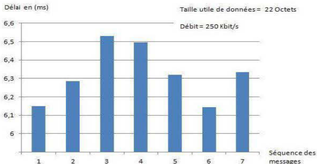
Figure 5. 9 : Délai de traitement au niveau de l'USRP
