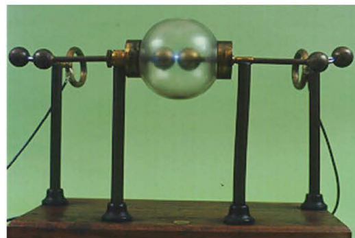
Figure 2 : Oscillateur de Righi
