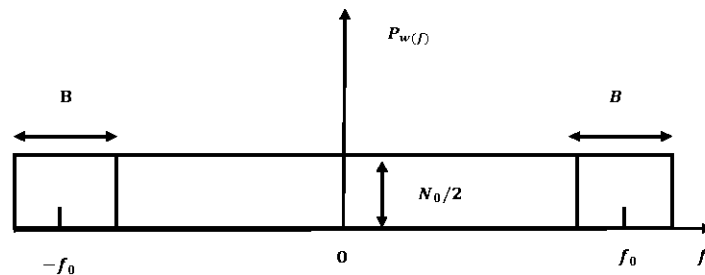
Figure 23 : Équivalence large bande de l'AWGN à bande limitée.
