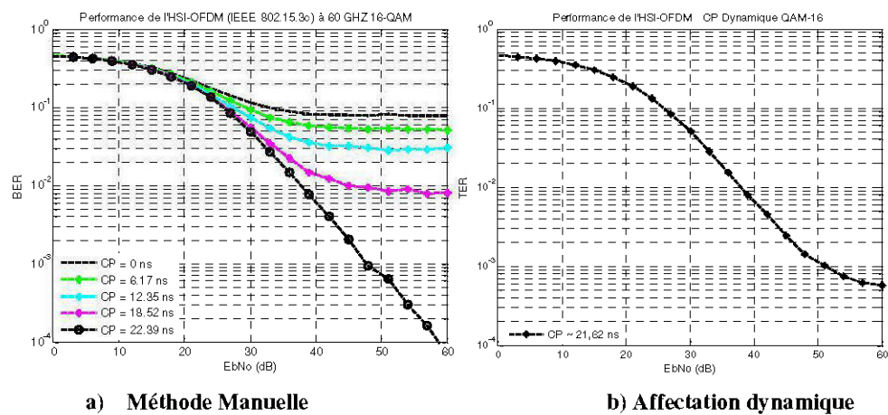
Figure 37 : TER OFDM 16-QAM dans le canal de Rice à 60 GHz Rms= 22 ns
