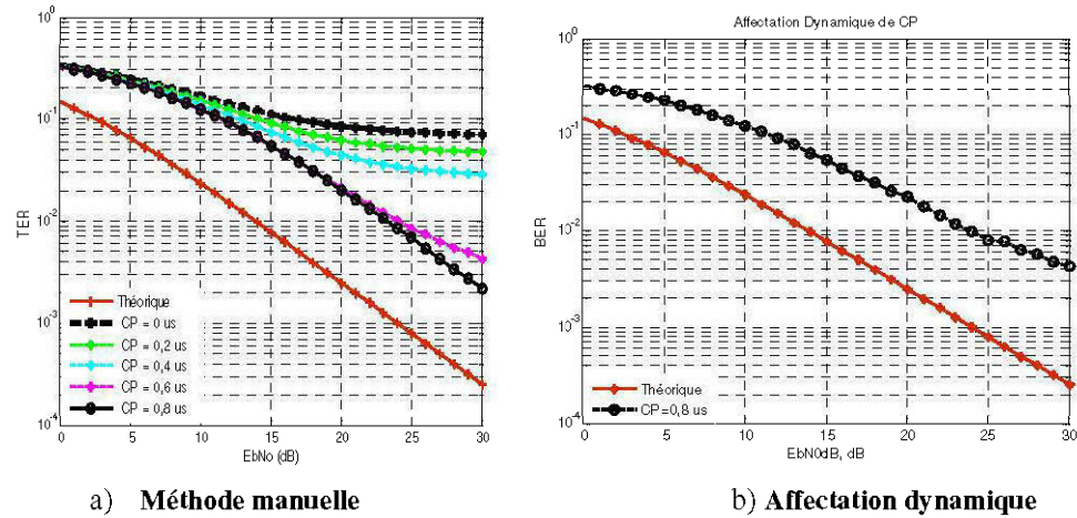
Figure 34: BER dans le canal de Rayleigh 16-QAM pour R_{ms}=0,8\mu s
