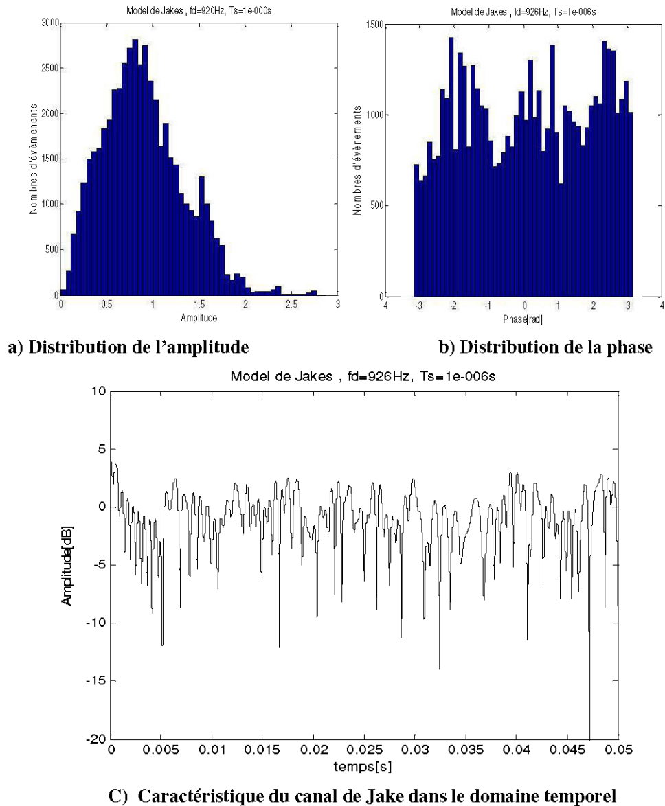
Figure 14 : Modèle de canal de Jake.
