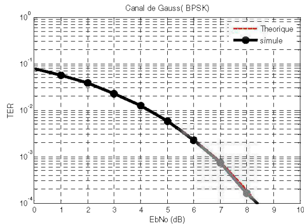
Figure 25: TER de l'OFDM BPSK dans un canal de Gauss
