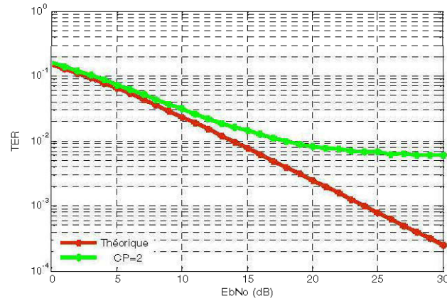
Figure 30 : Taux d'erreur binaire un canal de Rayleigh pour CP= 0,2 \mu s
