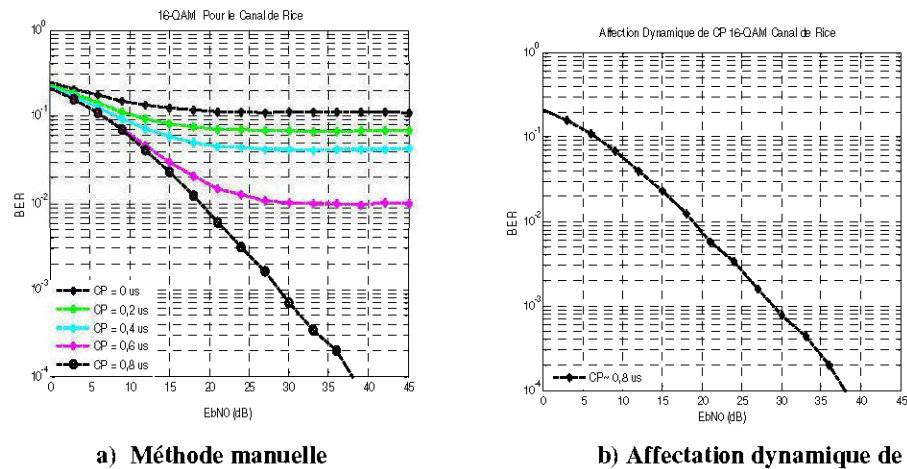
a) Méthode manuelle b) Affectation dynamique de CP Figure 27 : Performance de L'OFDM dans un Canal de Rice pour du 16-QAM Rms=0,8 \mu s
