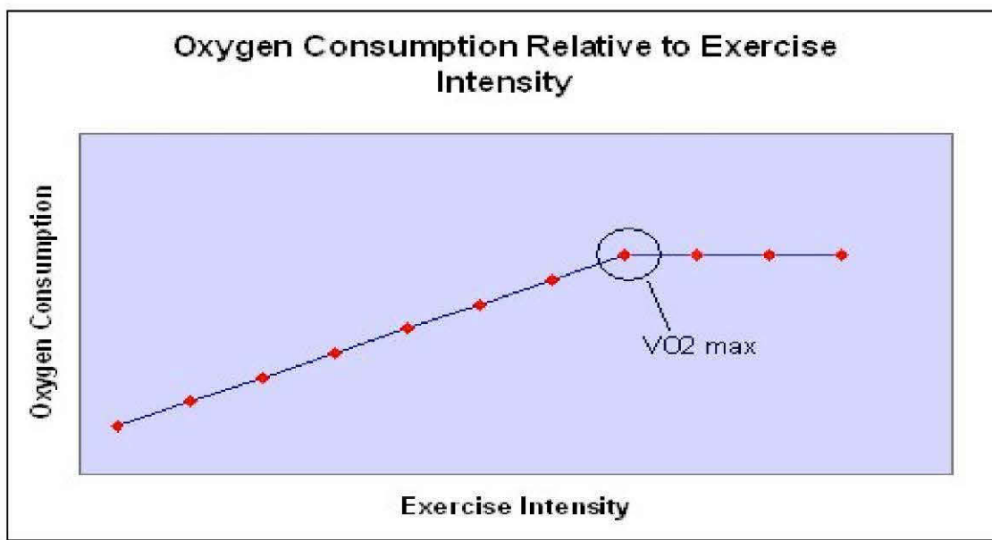
Figure 2. Consommation d'oxygène par rapport à l'intensité de l'exercice
