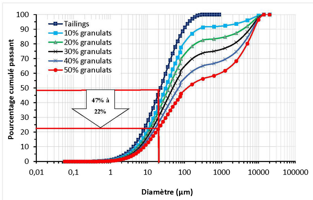
Figure 5.2 : Granulométrie des mélanges résidus-granulats B (0-20 mm)
