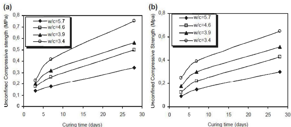
Figure 2.14 : Évolution de l'UCS en fonction du temps de cure pour des mélanges avec différents w/c (Kesimal et al., 2005)
