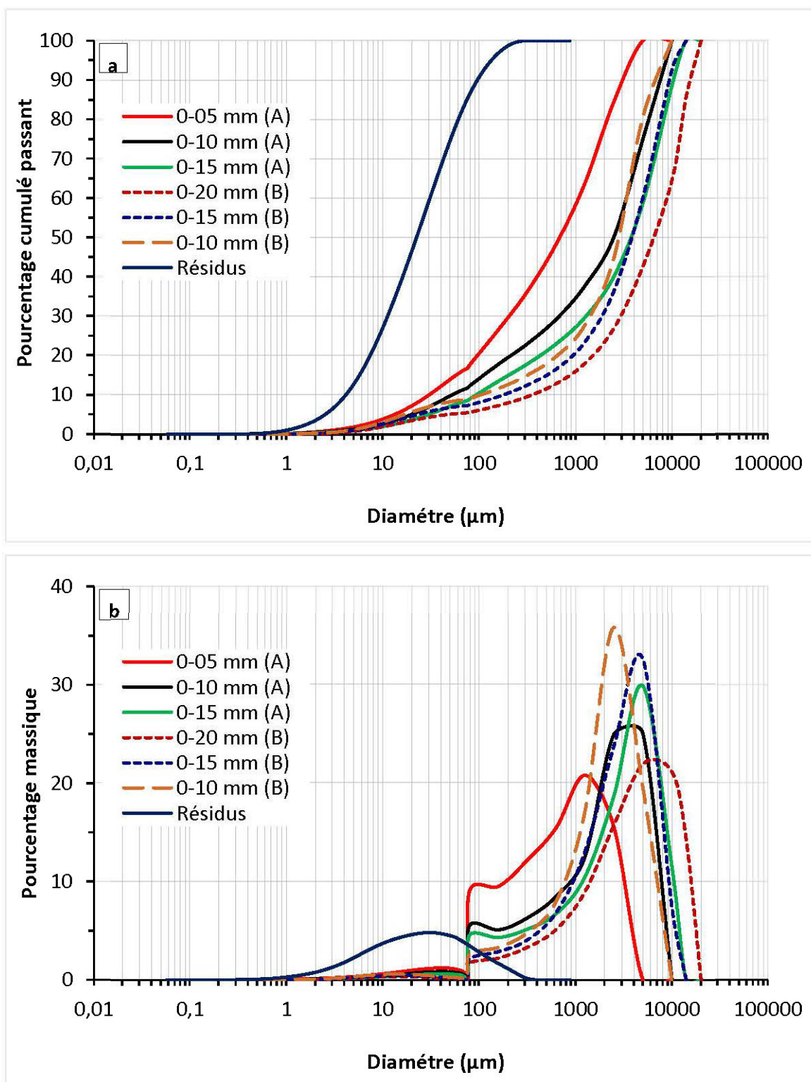
Figure 3.4 : Distributions granulométriques des résidus et des granules des stériles A et B : a) courbes cumulé, b) courbes incrémentales (histogrammes)
