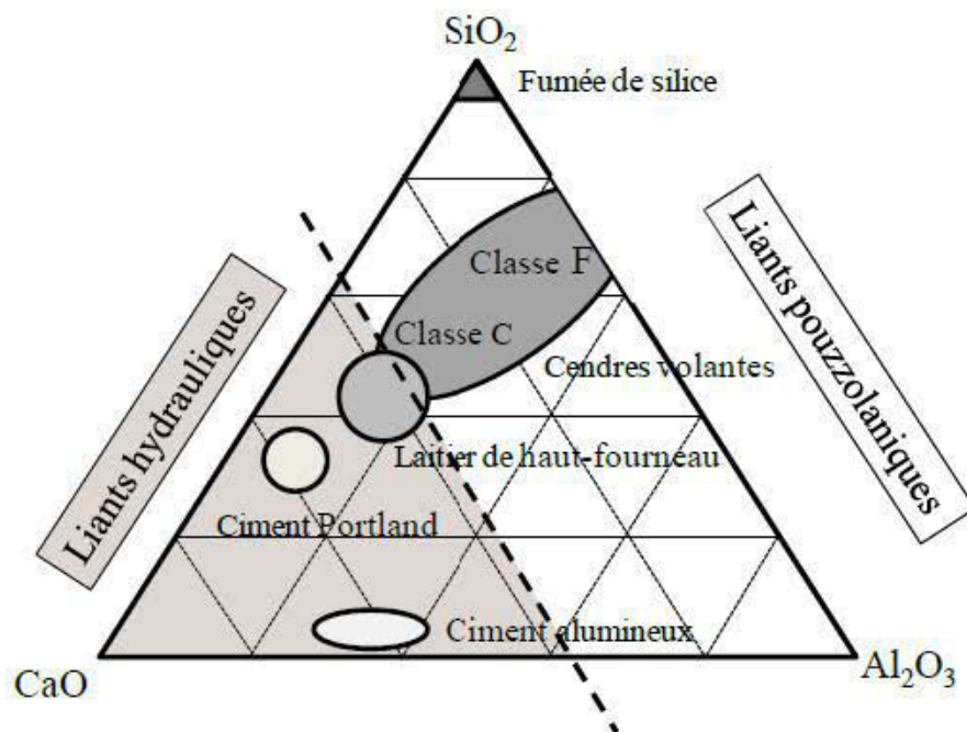
Figure 2.2 : Diagramme ternaire CaO-Al 2 O 3 -SiO 2 montrant la composition chimique de quelques liants hydrauliques et pouzzolaniques (Coussy, 2011)
