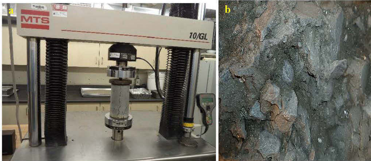
Figure 3.12 : Essai de compression uniaxiale sur un échantillon de remblai mixte (a) et vue intérieure du remblai après cassage (b)
