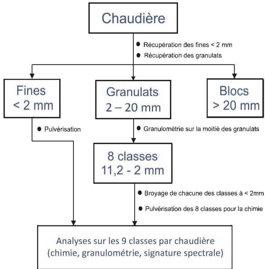
Figure 3.3: Organigramme de préparation des chaudières
