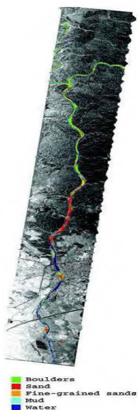
Figure 2.32 : Images Hymap de la rivière Odiel. On distingue trois parties distinctes. La première dominée par les galets, la seconde par le sable et la dernière par la vase. (Riaza et al. , 2012)
