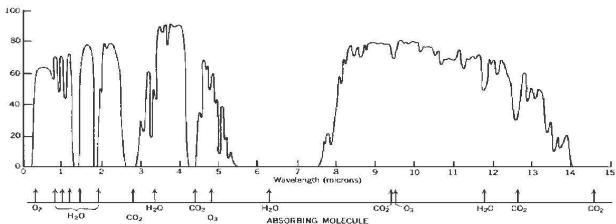
Figure 2.10 : Spectre d'absorption atmosphérique. L'aire compris en haut de la courbe correspond à l'énergie absorbée. (Lillesand et al. , 2015)
