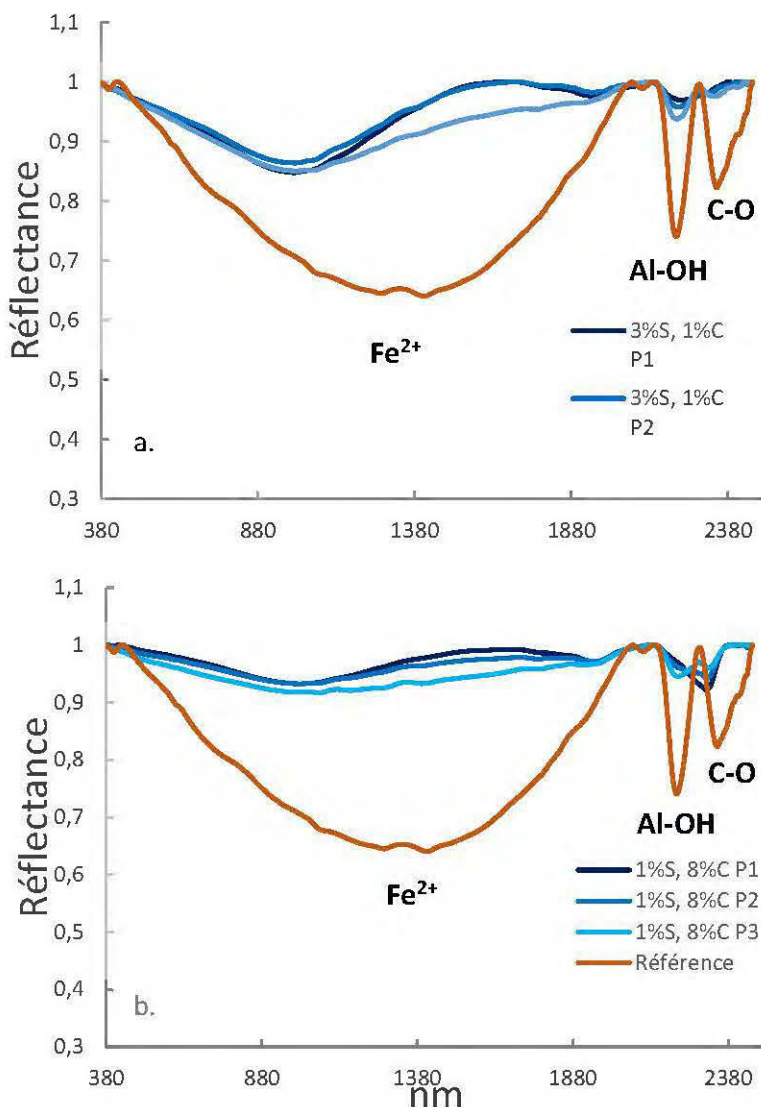
Figure 4.34 : Signature spectrale des poudres 3%S, 1%C (a.) et 1%S, 8%C (b.) vs signature du bloc référence
