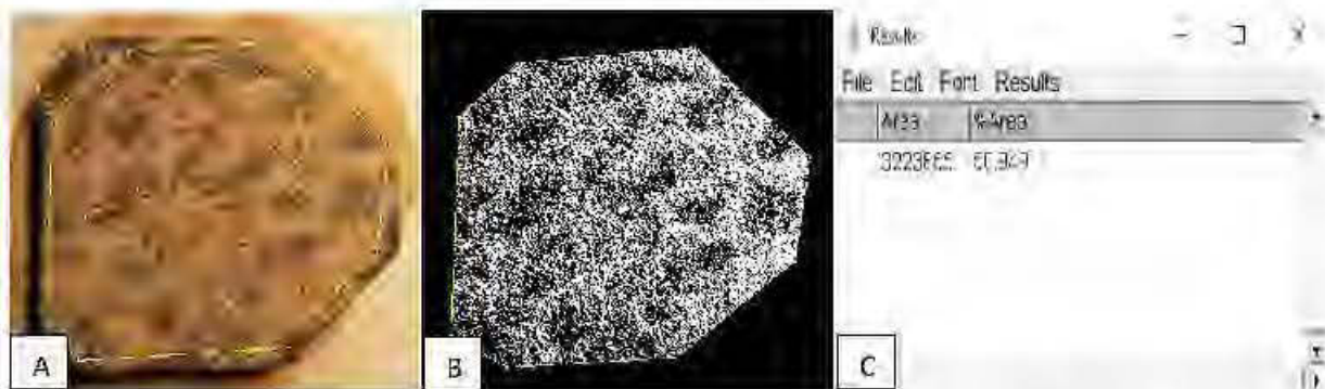
Figure 3.24 : Procédure complète d'analyse avec ImageJ pour l'échantillon 16-ZFA-6 (B3) P2. Détourage (A), image binaire (B), résultats (C)
