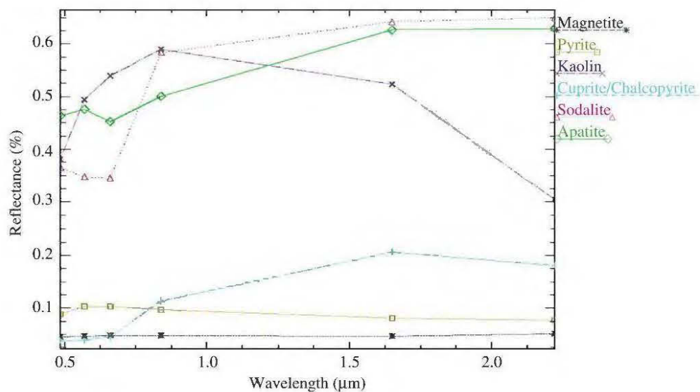
Figure 2.19 : Les différentes phases pures identifiées sur la scène étudiée. (Pal et al. , 2011)
