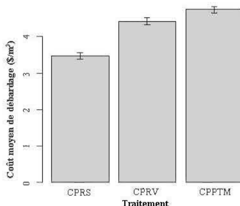
Figure 30 Coûts moyens de débardage ($/m 3 ) par traitement : CPRS, CPRV et CPPTM dans les secteurs d'étude ; et erreur type.
