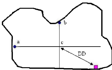
Figure A.2.6 Illustration de la méthode du centroïde de calcul de la distance moyenne de débardage (Koger et Webster, 1984) pour une bloc de récolte de forme irrégulière et débardage à jetée.
