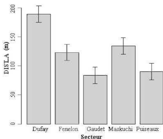
Figure 15 Distance de débarbage DIST_A moyenne par secteur d'étude : Dufay, Fénelon, Gaudet, Maskuchi et Puiseaux ; et erreur type .
