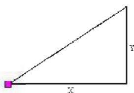
Figure A.2.3 Illustration de la méthode et équation de calcul de la distance moyenne de débardage de Suddarth (1952) pour une bloc de récolte de forme régulière (triangle rectangle) et débardage à jetée.
