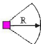
Figure A.2.2 Illustration de la méthode et équation de calcul de la distance moyenne de débardage de Suddarth (1952) pour une bloc de récolte de forme régulière (segment circulaire) et débardage à jetée.
