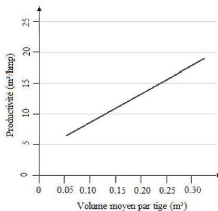
Figure 7 Productivité d'une abatteuse-façonneuse ( \text{m}^3/\text{hmp} ) en fonction du volume moyen par tige 6 ( \text{m}^3 ).
