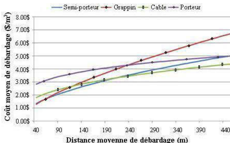
Figure A.1.6 Coûts moyens de débarbage ($/m 3 ) par type de débardeur utilisé : Semi-porteur, Grappin, Câble et Porteur, selon la distance de débarbage combinée considérant différents niveaux de rétention (pourcentage et configuration), position et concentration du volume.
