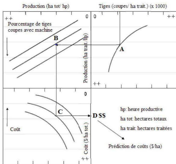
Figure 8 Nombre de tiges récoltées (coupes/ ha traités) en fonction de la production (ha tot/hp) et les coûts de récolte 7 ($/ha tot). (A) nombre de tiges en fonction de la productivité (B) pourcentage de tiges en fonction de la productivité (C) coûts de récolte en fonction de la productivité.
