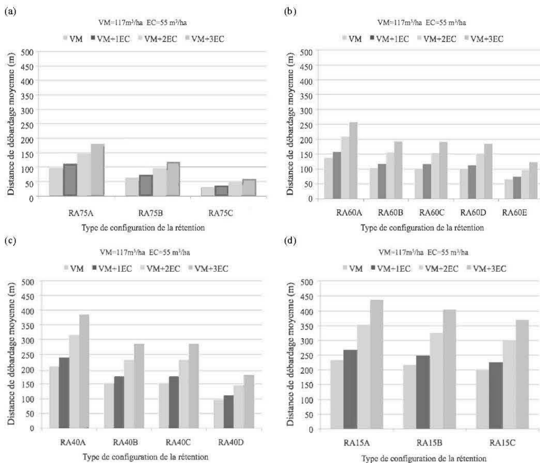
Figure A.1.5 Distance moyenne de débardage combinée en fonction du volume à extraire : VM, VM+1EC, VM+ 2EC et VM+3EC (volume moyen et volume moyen plus un, deux et trois écarts-type) et types de configuration de la rétention : (a) RA75A, RA75B et RA75C, (b) RA60A, RA60B, RA60C, RA60D et RA60E, (c) RA40A, RA40B, RA40C et RA40D et (d) RA15A, RA15B et RA15C. (RA) rétention agglomérée, (75, 60, 40 et 15) pourcentages de rétention et (A, B, C, D ou E) configurations de la rétention.
