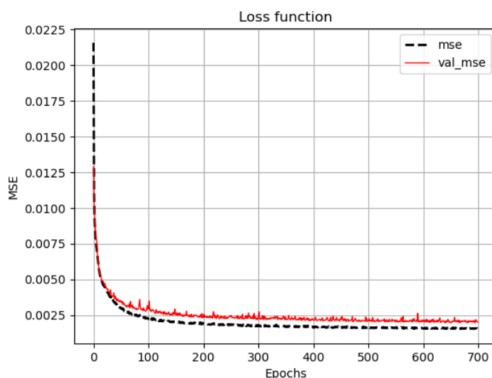
Figure 4-23 Évolution de la fonction perte du DNN (MSE) en fonction de nombre d'itérations
