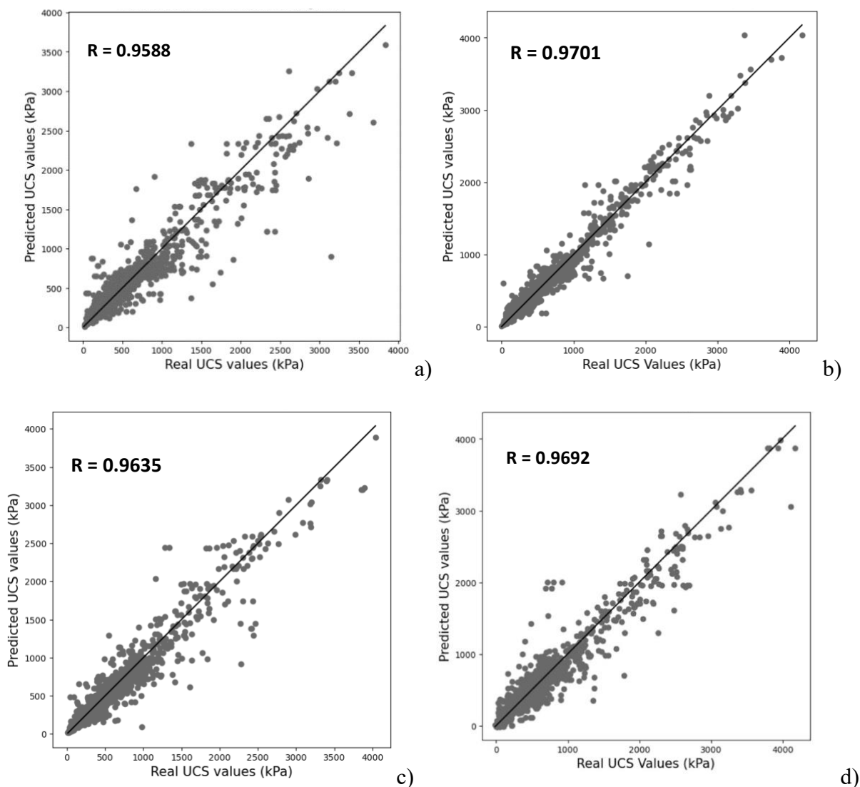
Figure 4-19 Comparaison sur la pente 1 :1 des prédictions des modèles; a) RF, b) GBR, c) XGBR, d) DNN
