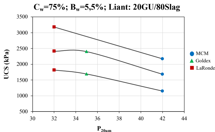
Figure 4-7 Variation de l'UCS en fonction de P_{20\mu m} des résidus
