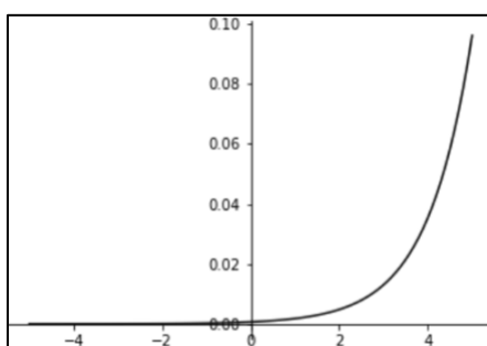
Figure 3-16 Fonction d'activation Softmax (Farhadi, 2017)
