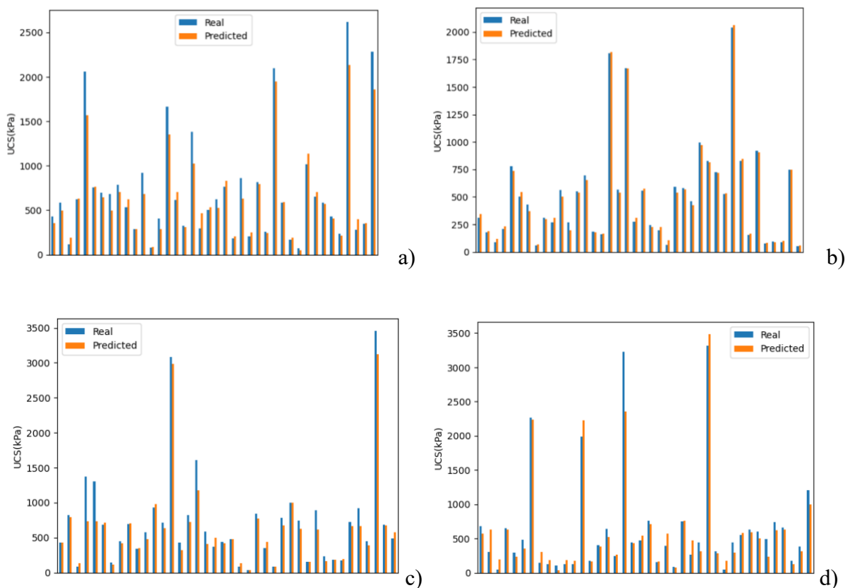
Figure 4-24 Comparaison des valeurs de l'UCS dans l'ensemble de données du test et celles prédites par les modèles; a) RF, b) GBR, c) XGBR, d) DNN
