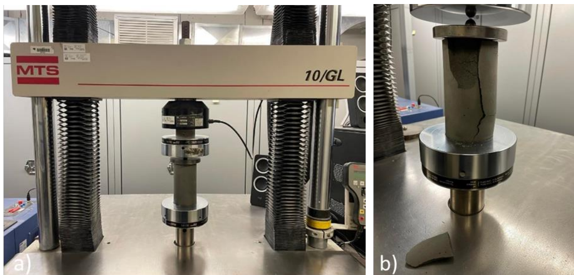
Figure 3-8 Essai de compression uniaxiale : a) presse mécanique rigide MTS 10/GL ; (b) échantillon cassé après l'essai
