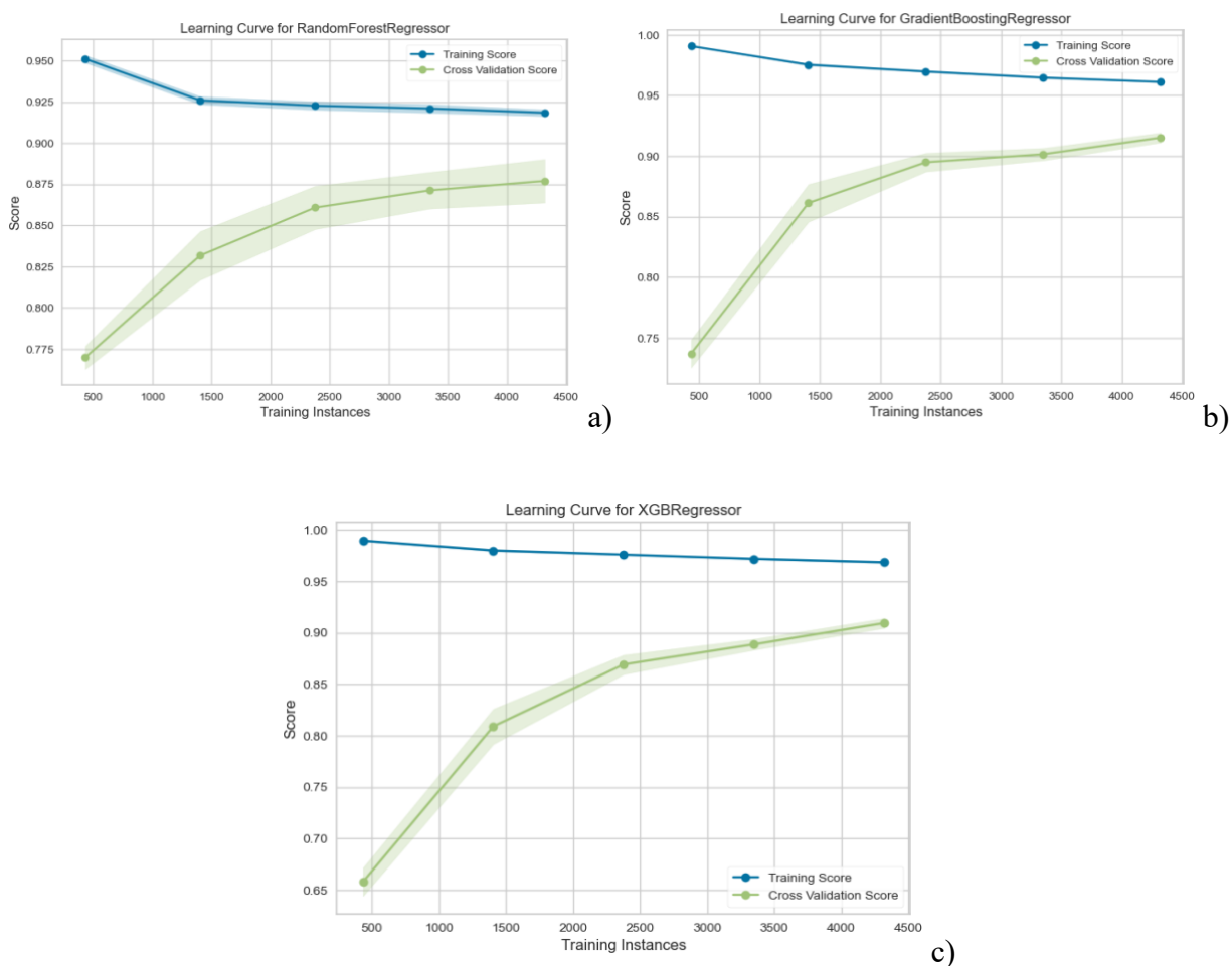
Figure 4-21 Courbe d'apprentissage des modèles : a) RF, b) GBR, c) XGBR
