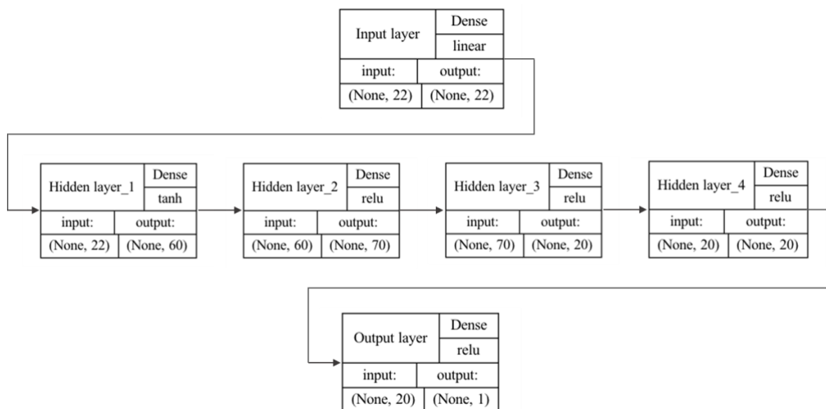
Figure 4-18 Description des couches du DNN
