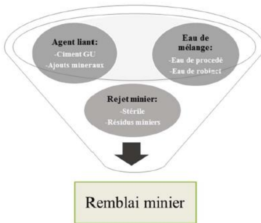
Figure 1-1 Principaux ingrédients d'un remblai minier cimenté
