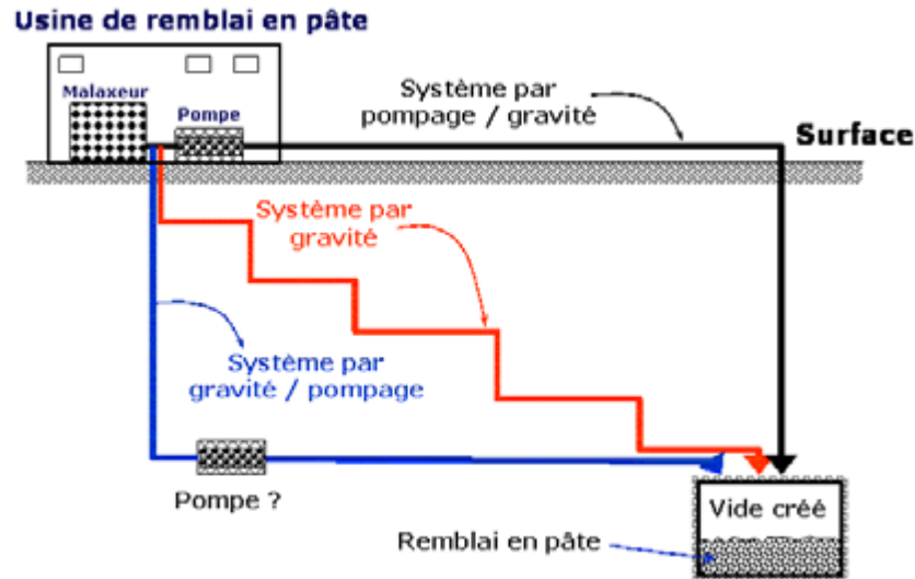
Figure 2-5 Différents systèmes de distribution des remblais sous terre (Belem and Benzaazoua, 2003a)
