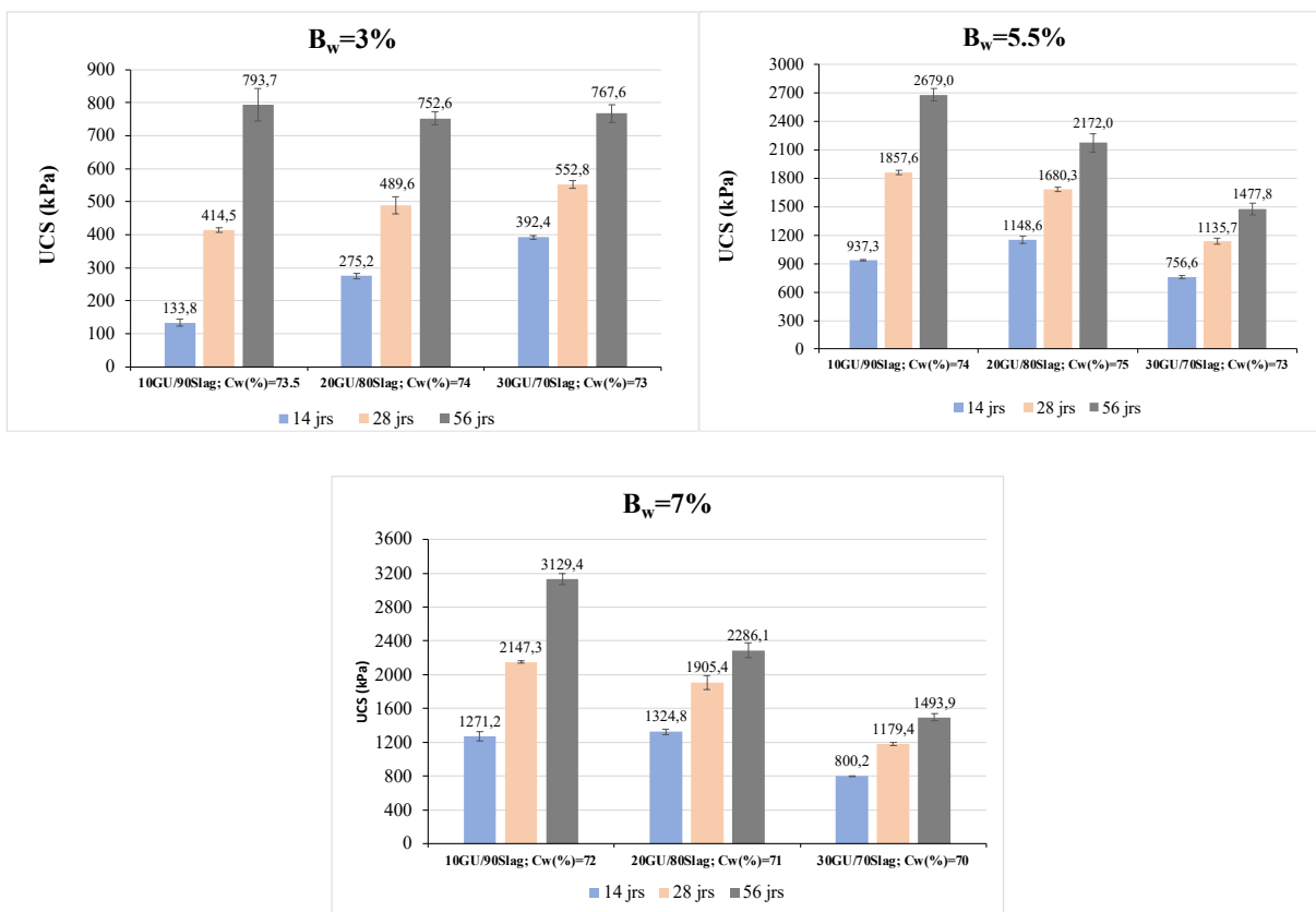
Figure B-3 Évolution de l'UCS en fonction de la formulation de liant GU/Slag
