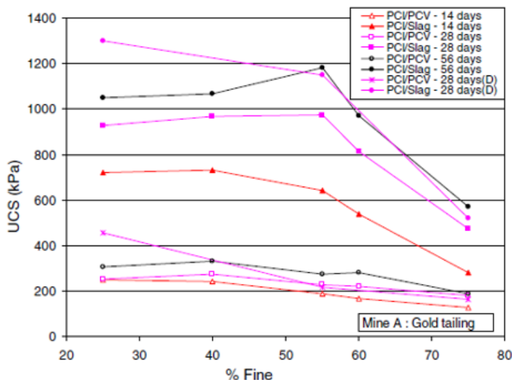
Figure 2-7 Influence des particules fines ( d < 20 \mu\text{m} ) sur l'UCS (Fall et al., 2004)
