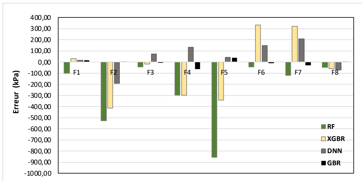
Figure 4-27 Erreurs de prédiction des modèles
