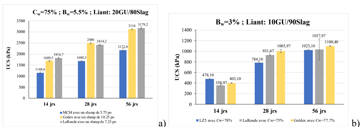
Figure 4-6 Variation de l'UCS selon le type de résidus
