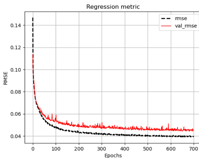
Figure 4-22 Évolution de la métrique du DNN (RMSE) en fonction de nombre d'itérations
