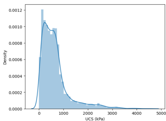
Figure 4-11 Densité de probabilité de l'UCS
