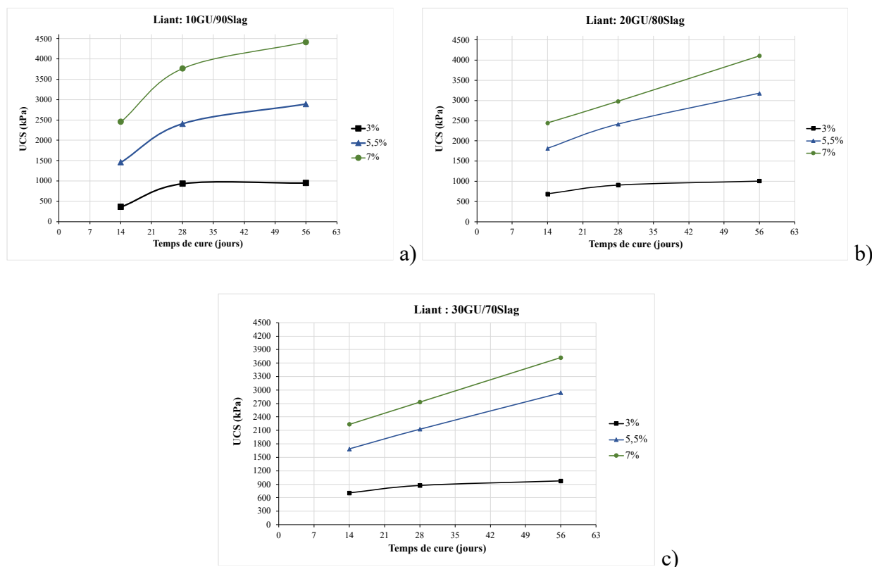
Figure 4-5 Variation de l'UCS en fonction de temps et pourcentage de liant avec les résidus de LaRonde
