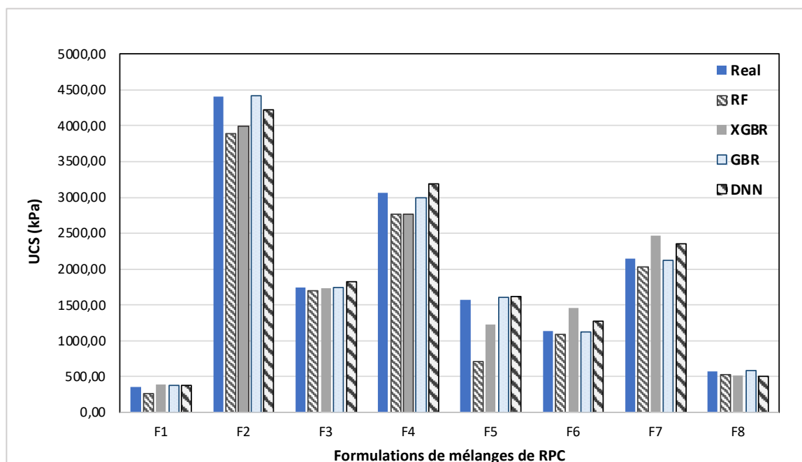
Figure 4-26 Comparaison des UCS prédites par les modèles et celles obtenues expérimentalement
