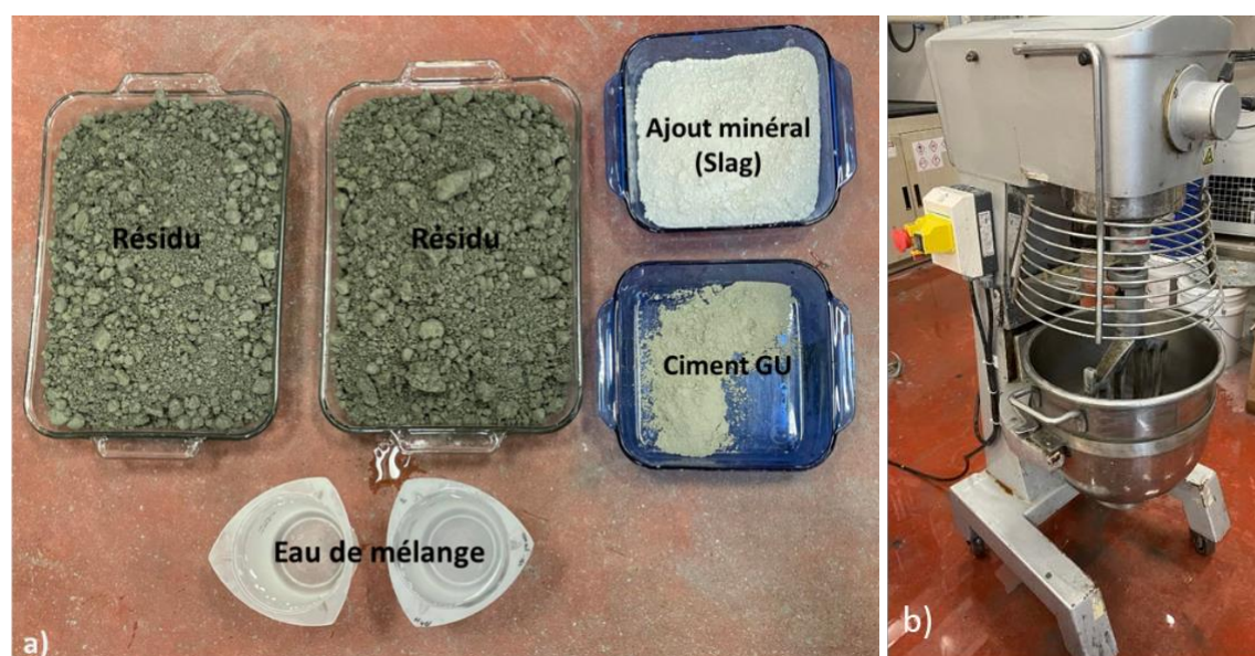
Figure 3-5 Préparation des mélanges : a) les ingrédients de RPC; b) mélangeur Hobart
