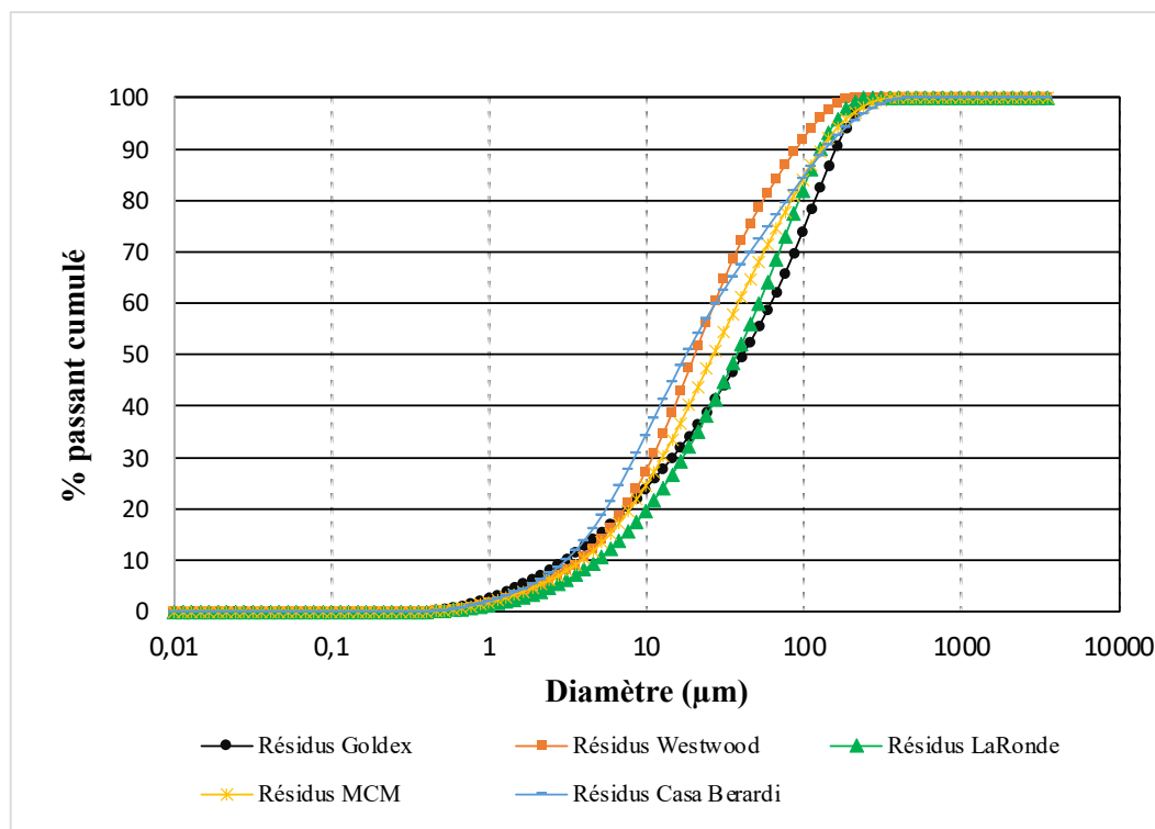
Figure 4-1 Courbes granulométriques des résidus testés
