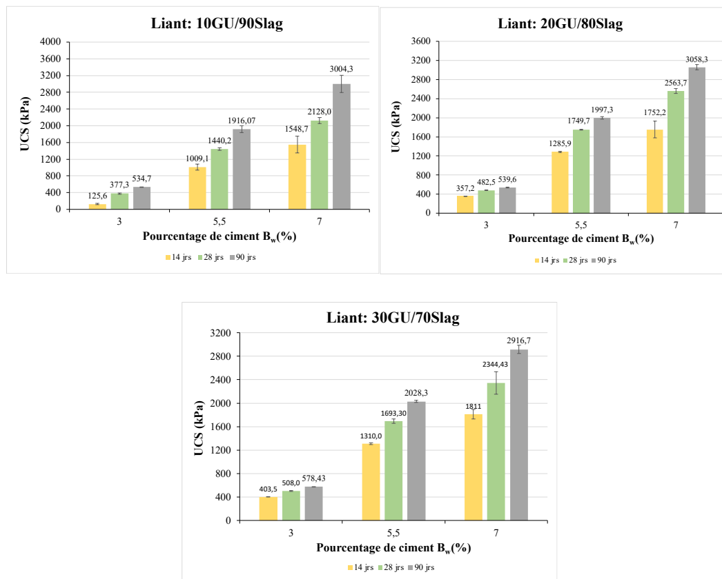
Figure B-4 Évolution de l'UCS en fonction du B_w (%) et temps de cure
