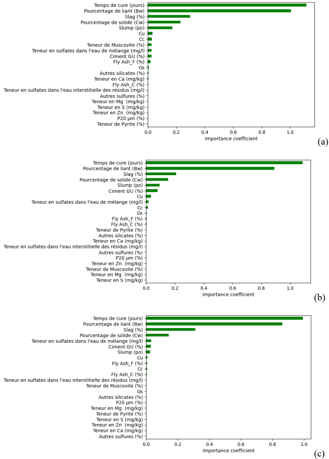
Figure 4-25 Importance des variables sélectionnées par les modèles : (a) GBR, (b) XGBR, (c) RF
