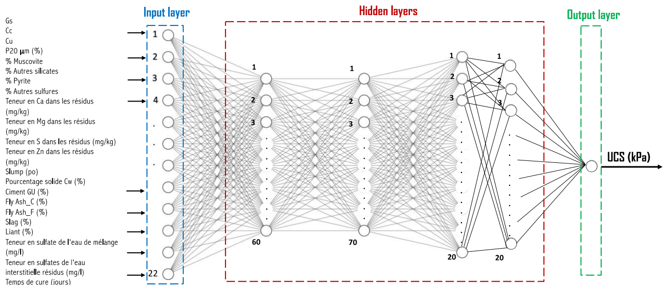
Figure 4-17 Architecture du réseau Deep Neural Network (DNN)
