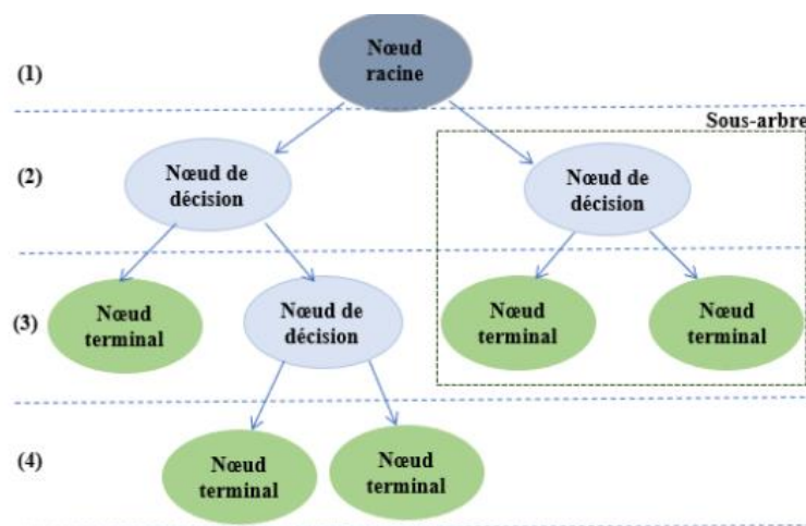
Figure 3-10 Structure d'un arbre décisionnel
