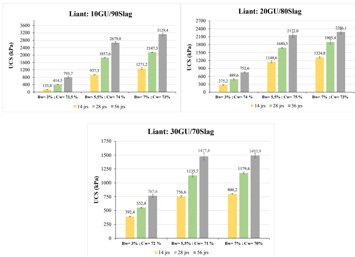
Figure B-6 Évolution de l'UCS en fonction du B w (%) et du temps de cure
