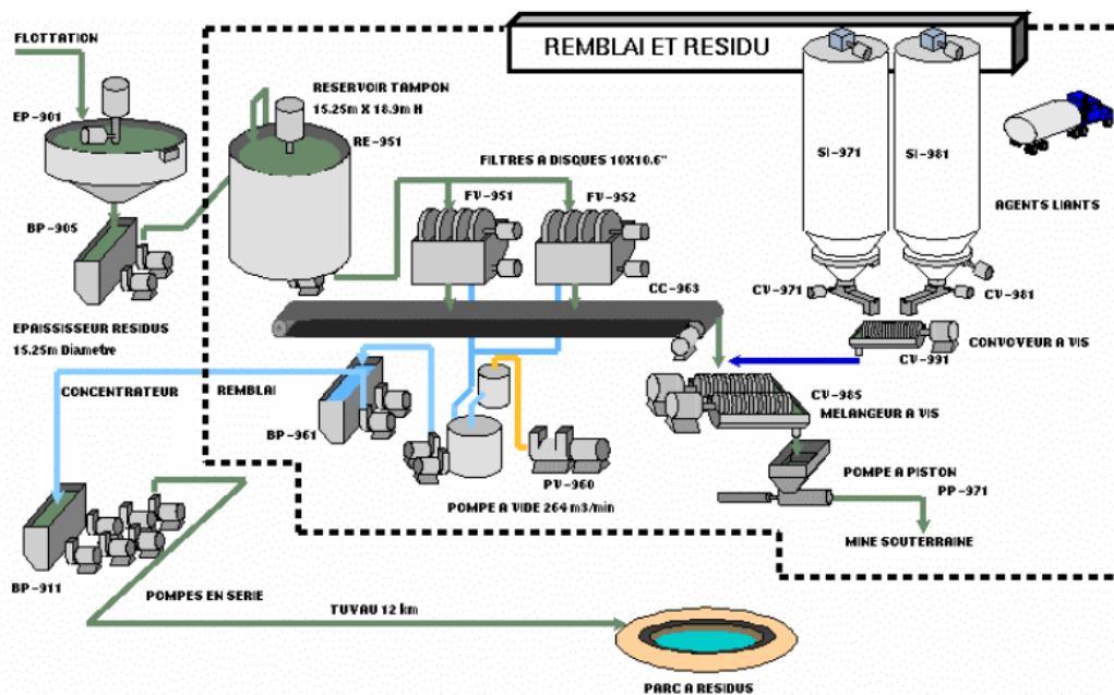
Figure 2-4 Schéma typique de la procédure complète de fabrication du remblai en pâte cimenté à l'usine (Belem and Benzaazoua, 2003a)
