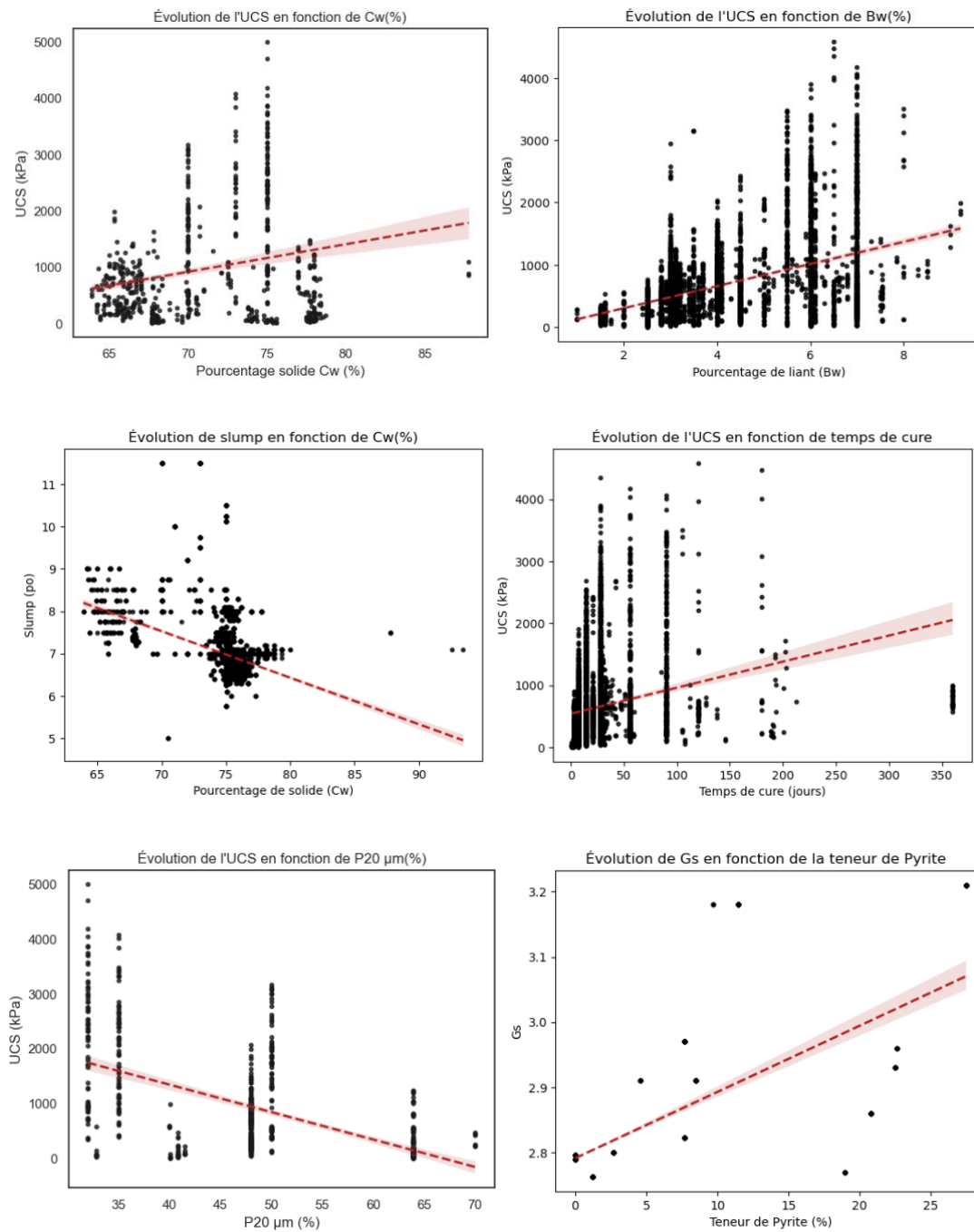
Figure 4-13 Tendances entre les variables
