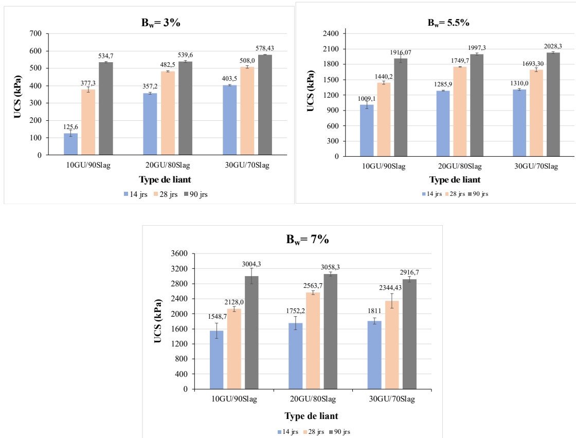
Figure B-1 Évolution de l'UCS en fonction de la formulation de liant GU/Slag
