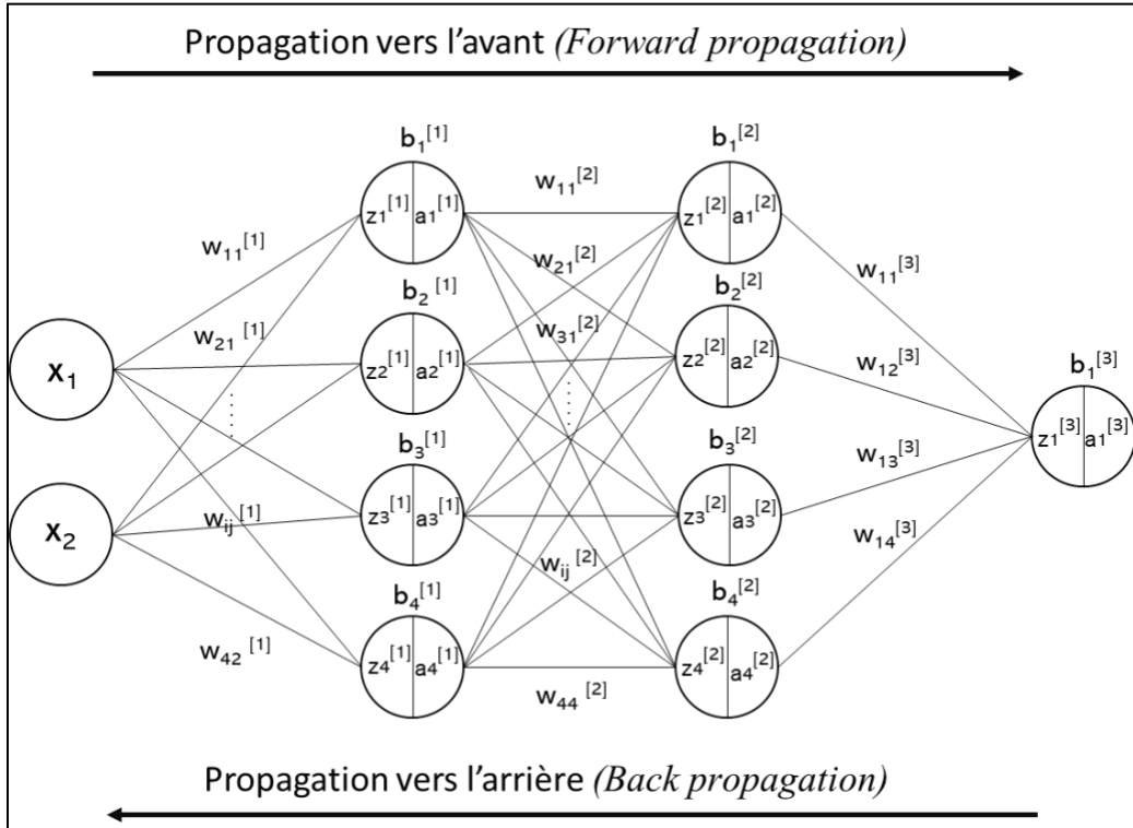
Figure 3-13 Réseau de neurones à rétropropagation vers l'arrière ( Feed-Forward Back Propagation Network-FFBPN )
