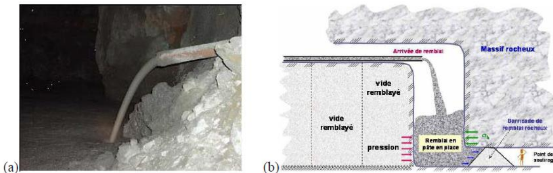
Figure 2-6 Mise en place du remblai : a) vide en cours de remblayage; b) schéma des composantes d'un vide remblayé (Belem and Benzaazoua, 2003a)
