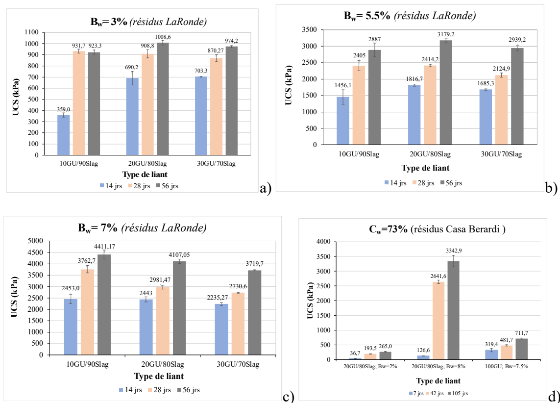
Figure 4-4 Variation de l'UCS selon le type de liant GU/Slag
