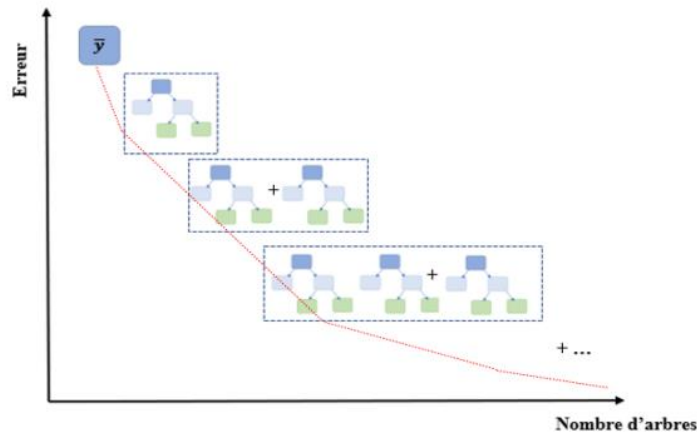
Figure 3-11 Évolution de l'erreur en fonction de nombre d'arbres
