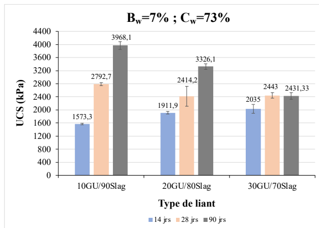
Figure B-2 Évolution de l'UCS en fonction de la formulation de liant GU/Slag
