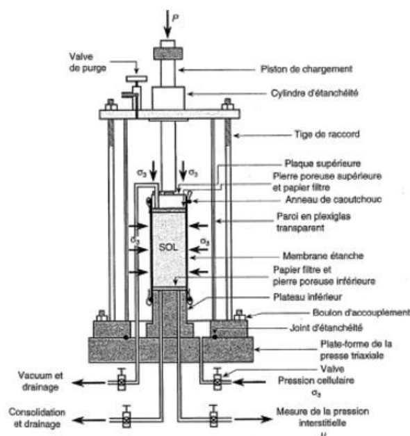
Figure 2-10 Appareil triaxial (Robitaille et Tremblay, 1997)
