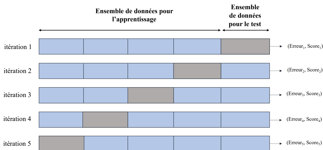
Figure 4-20 Schéma du processus de validation croisée
