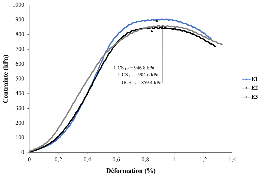
Figure 4-2 Courbes contrainte-déformation pour le mélange 30GU/70Slag à 3% liant avec les résidus de LaRonde et à 28 jours de cure
