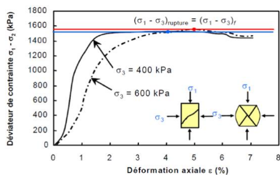
Figure 2-11 Courbe typique d'essais en compression triaxiale sur des remblais en pâte (Belem, 2022 ; Notes de cours)
