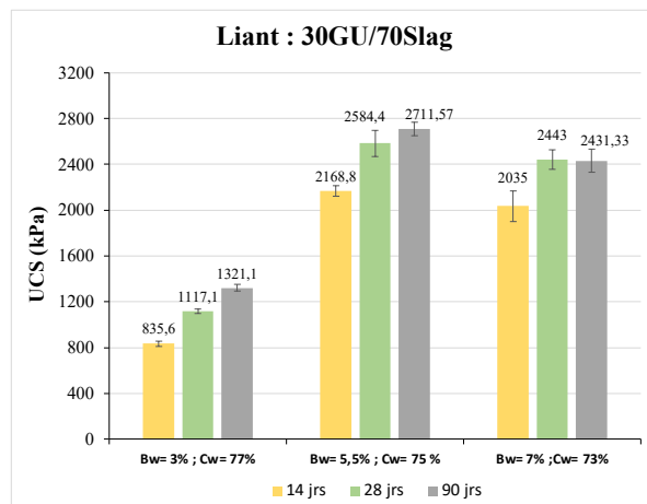
Figure B-5 Évolution de l'UCS en fonction du B w (%) et temps de cure
