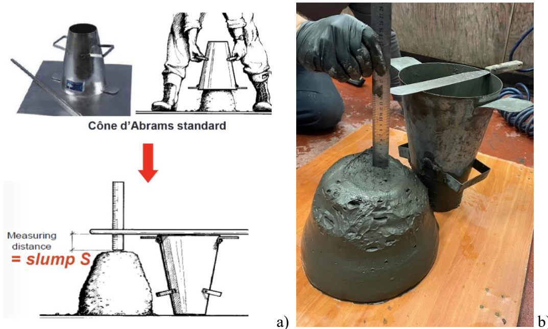
Figure 3-6 Mesure de l'affaissement à l'aide de la méthode standard du cône d'Abrams; a) au laboratoire, b) principe de mesure de l'affaissement
