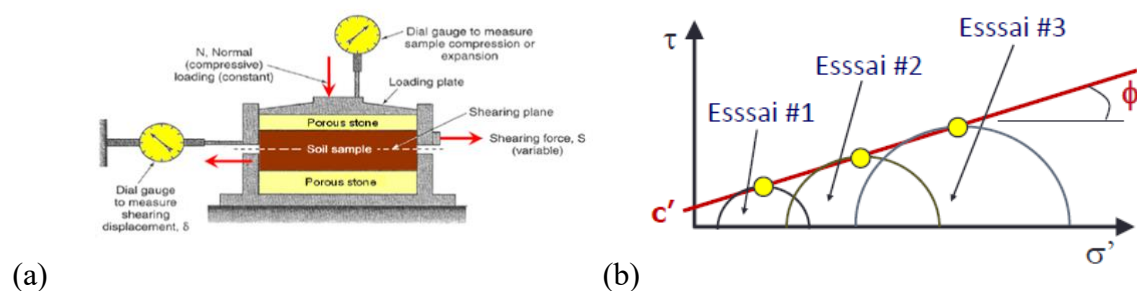
Figure 2-12 (a) Schéma d'une machine de cisaillement direct (McCarthy, 2010), (b) Enveloppe de rupture avec cohésion (Belem, 2022; Notes de cours)
