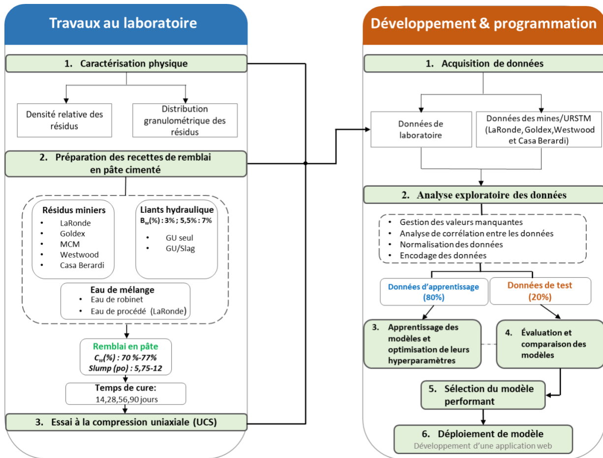
Figure 3-3 Démarche méthodologique générale de l'étude
