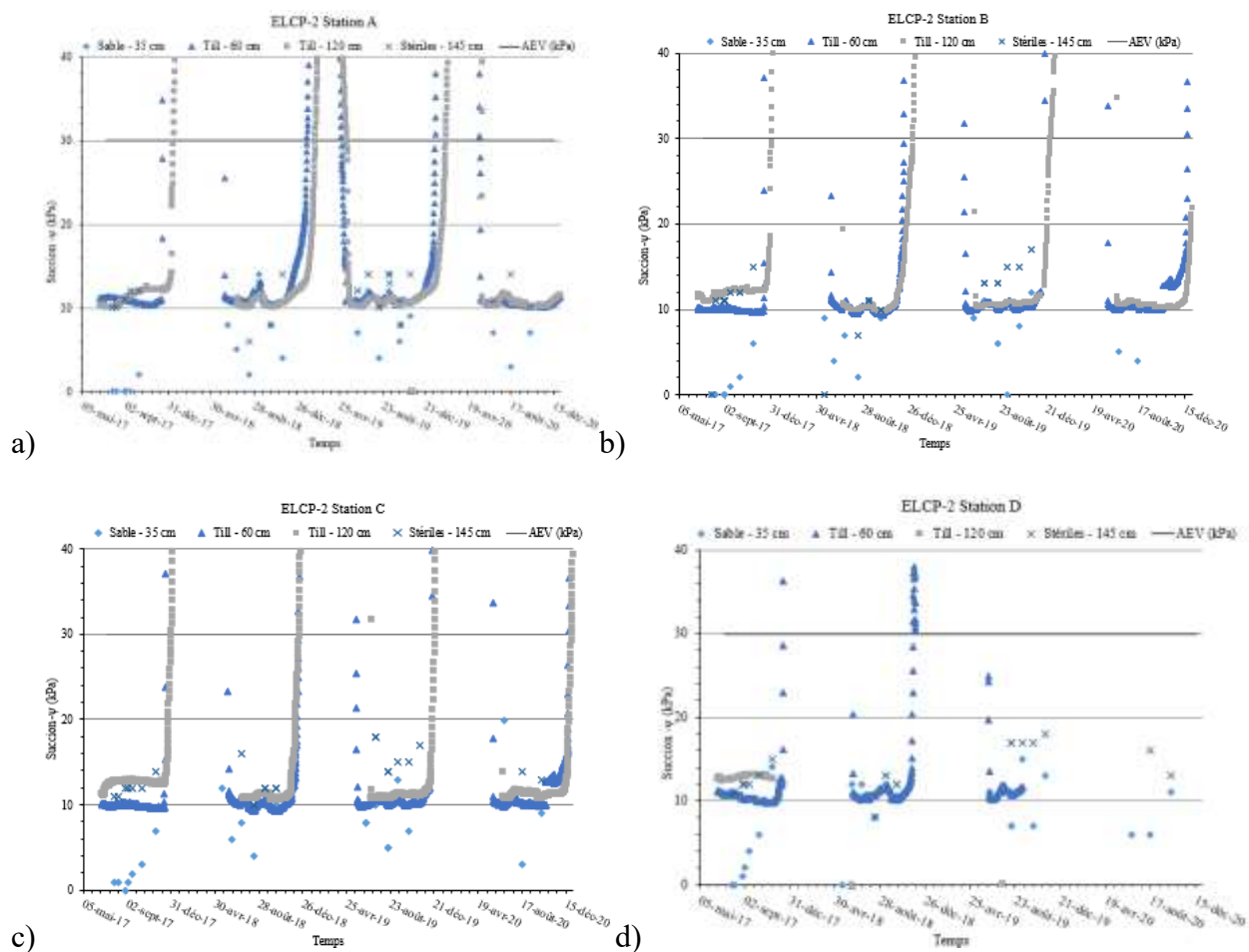
Figure 4.9 Résultats de l'évolution de la succion dans la cellule ELCP-2 : a) Station A, b) Station B, c) Station C, d) Station D.
