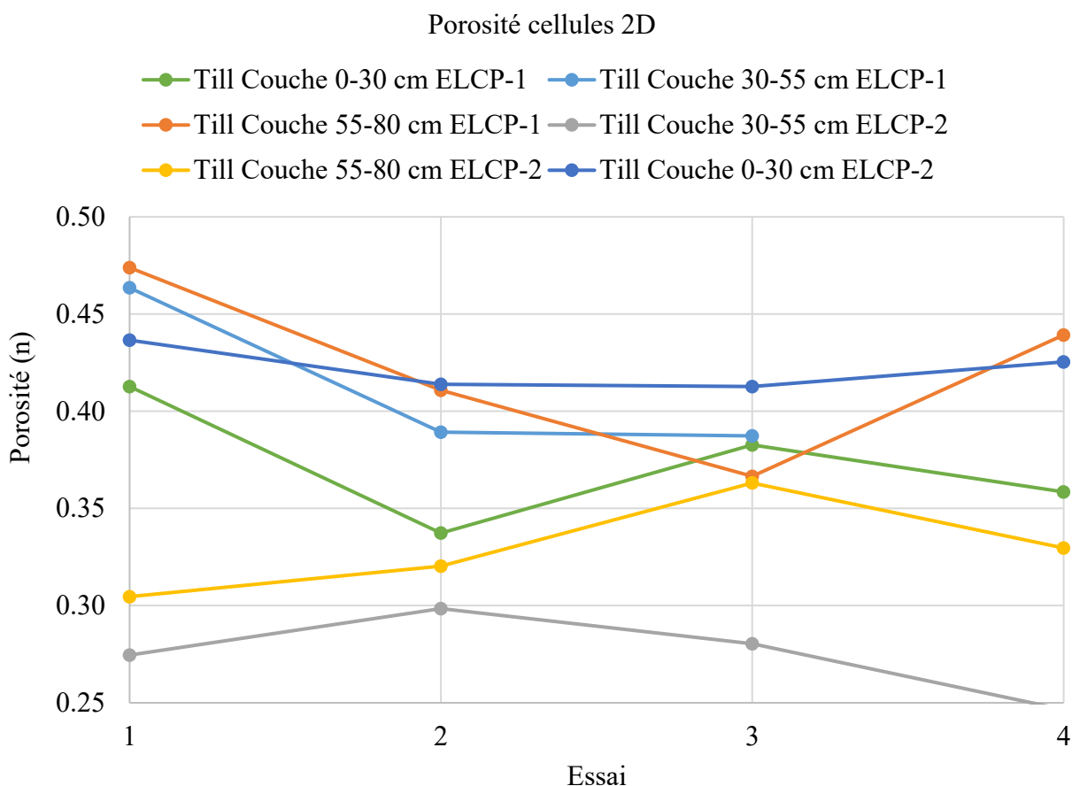
Figure 3.16 Résultats des mesures de porosité pour le till.
