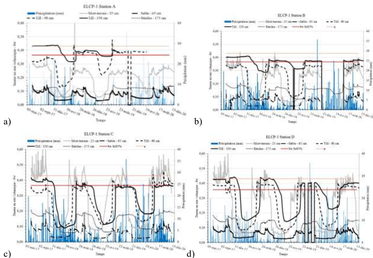
Figure 4.6 Résultats de l'évolution de la teneur en eau volumique ( \theta_w ) dans la cellule ELCP-1 : a) Station A, b) Station B, c) Station C, d) Station D.
