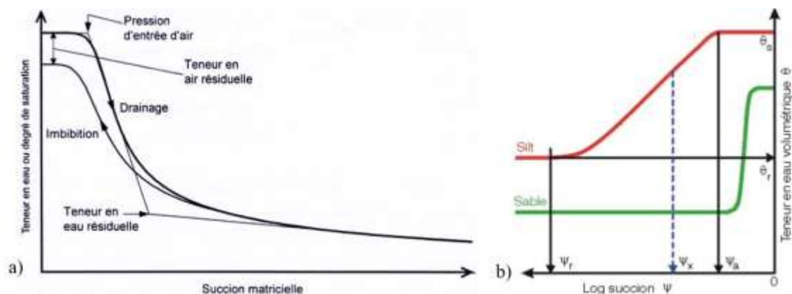
Figure 2.10 Courbe de rétention d'eau (CRE). a) Schéma du comportement d'une CRE. b) Comportement de la CRE pour différents types de sol. (Côté, 1998; Aubertin et al., 2002).
