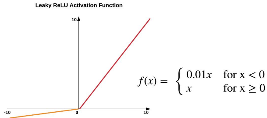
Figure 27 : fonction Leaky ReLU
