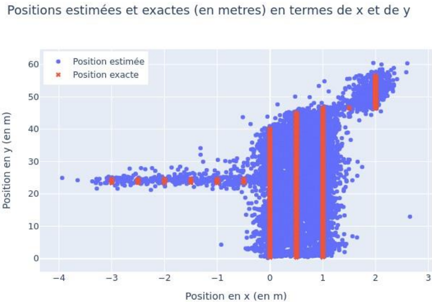
Figure 44: Visualisation des positions estimées et exactes dans le plan xy en utilisant TF
