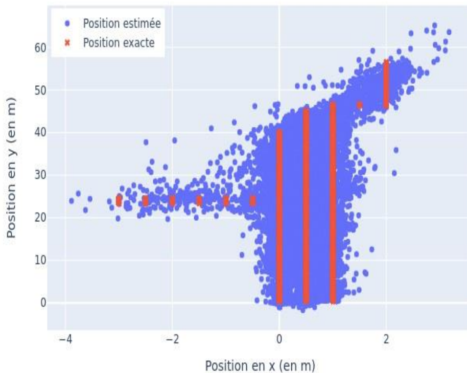
Figure 48: Visualisation des positions estimées et exactes dans le plan xy en utilisant Sc-L
