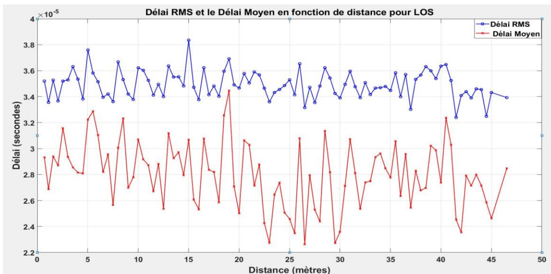
Figure 18 : Décreté RMS et décreté moyen en fonction de distance pour ligne de visée
