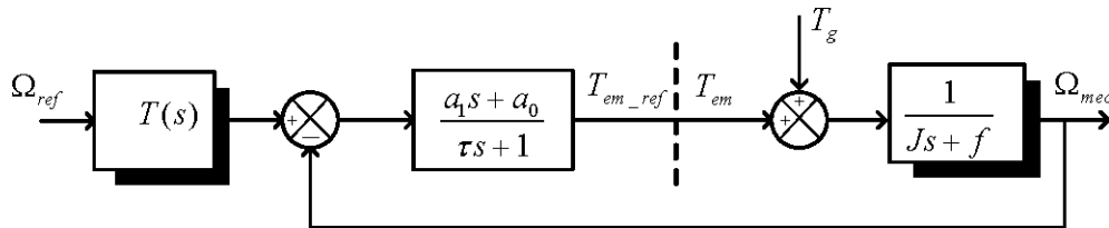
Figure 3-9 : Schéma bloc du correcteur PI à avance de phase
