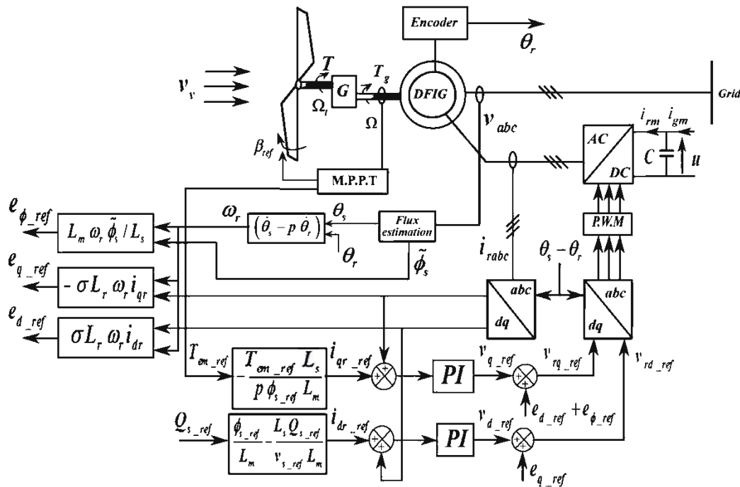
Figure 5-2 : Schéma-bloc du contrôle de la MADA
