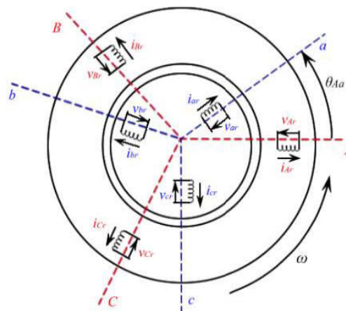
Figure 4-2 : Inductances du stator et inductances du rotor d'une machine asynchrone à double alimentation
