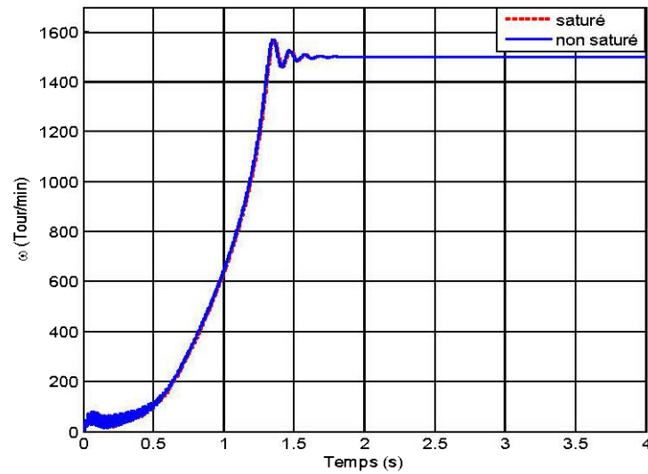
Figure 4-13: Comparaison vitesse du modèle saturé avec le modèle non saturé
