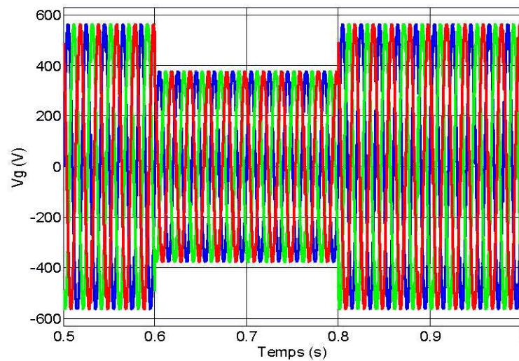
Figure 6-5 : Tension réseau durant un défaut triphasé.
