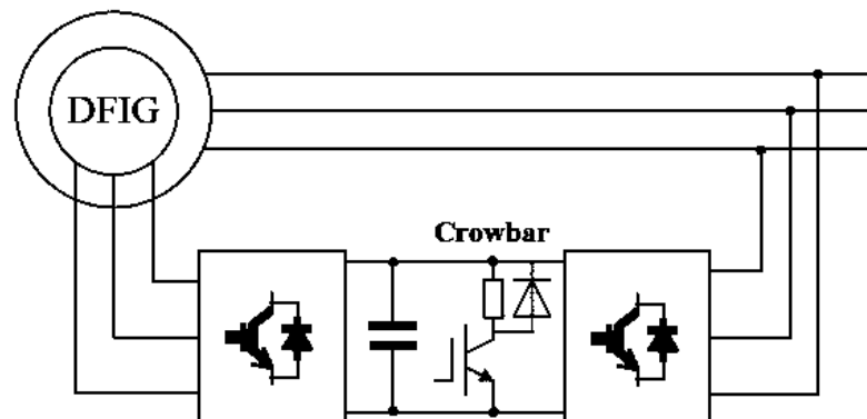
Figure 7-3 : Circuit de limitation de tension du bus continu
