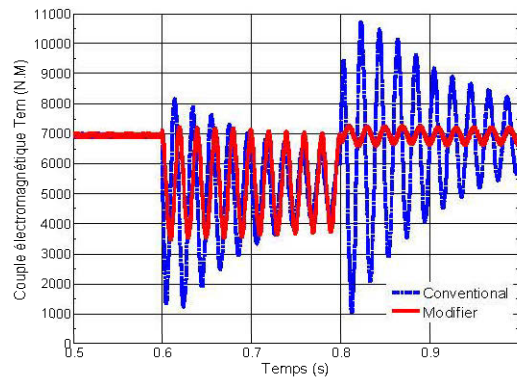
Figure 6-8 : Couple électromagnétique durant un creux de tension.
