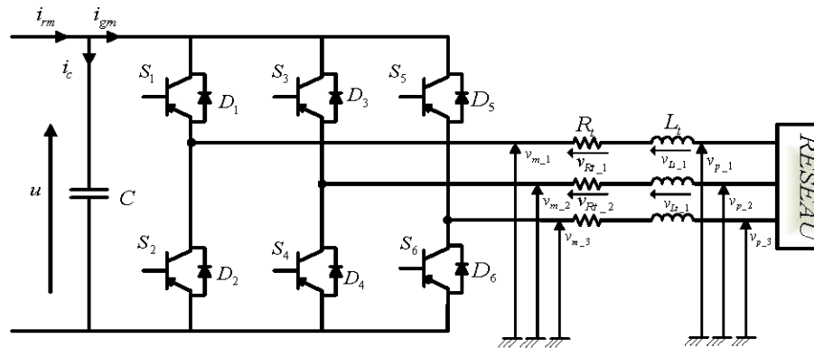
Figure 4-15 : Schéma électrique de la liaison au réseau via un convertisseur MLI
