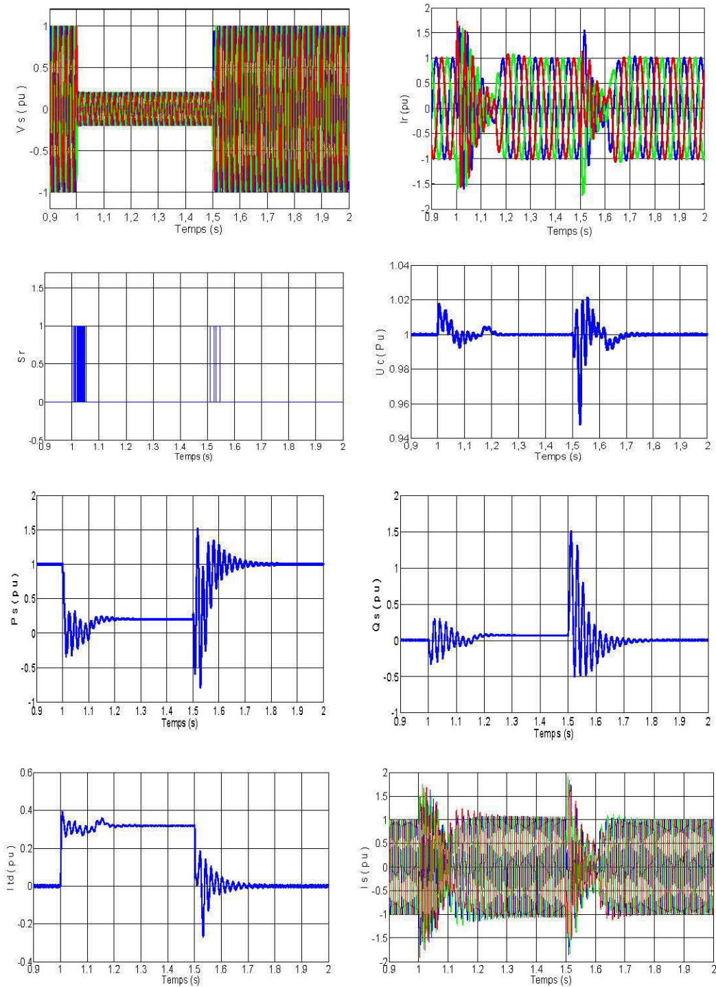
Figure 7-7 : Résultats de simulation pour une chute de tension de 80% pendant 0.5s
