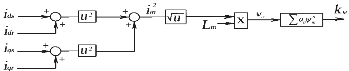
Figure 4-7 : Détermination de degré de saturation
