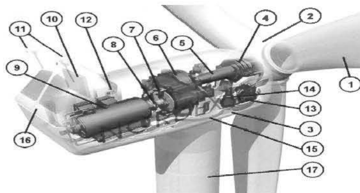
Figure 2-6 : Constitution de la nacelle
