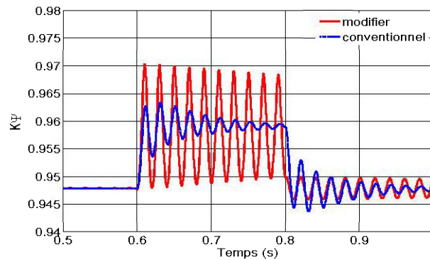
Figure 6-10 : facteur de saturation pendant un creux de tension
