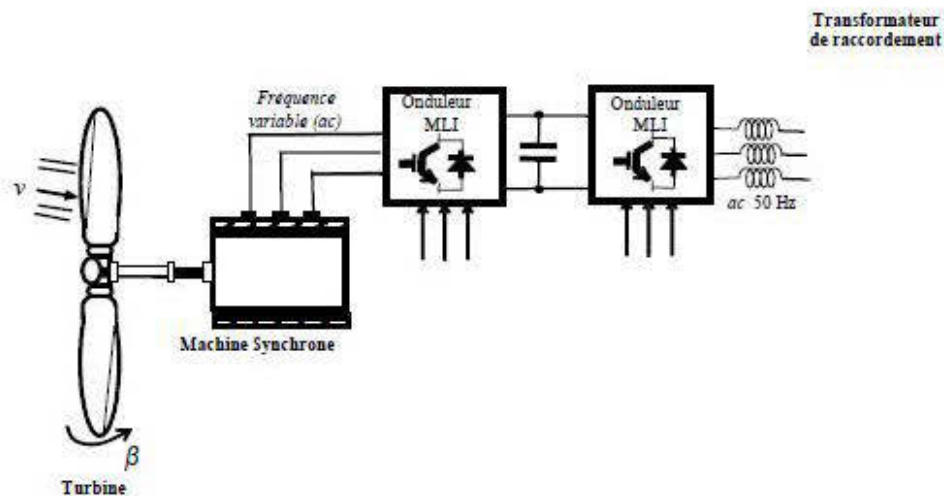
Figure 2-15 : Éolienne à vitesse variable basée sur une machine synchrone à grand nombre de paires de pôles
