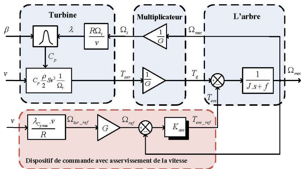
Figure 3-7 : Schéma bloc de la maximisation de la puissance extraite avec asservissement de la vitesse
