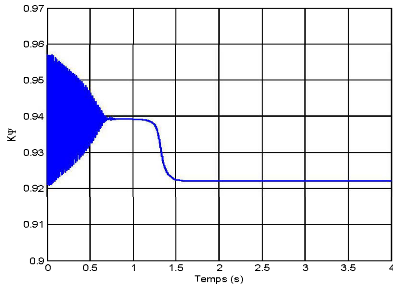
Figure 4-14 : Facteur de saturation K_{\psi}
