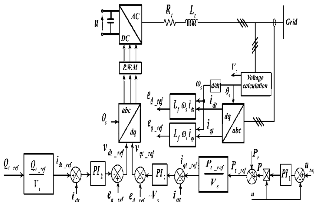
Figure 5-4 : Schéma-bloc du contrôle du convertisseur coté réseau
