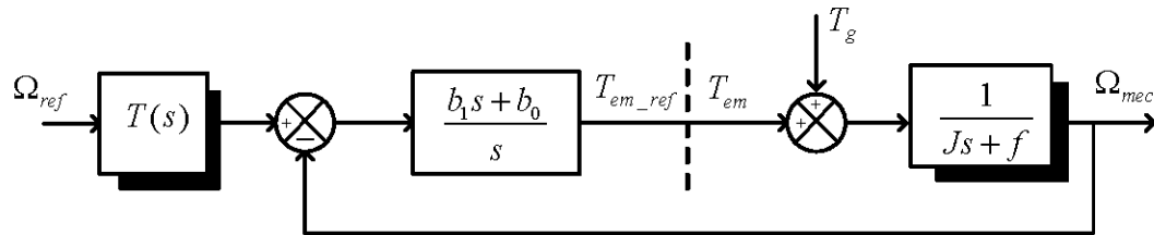
Figure 3-10 : Schéma bloc du correcteur PI avec anticipation
