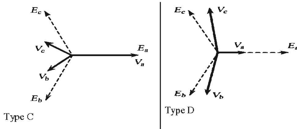
Figure 6-3 : Types de creux de tension de base
