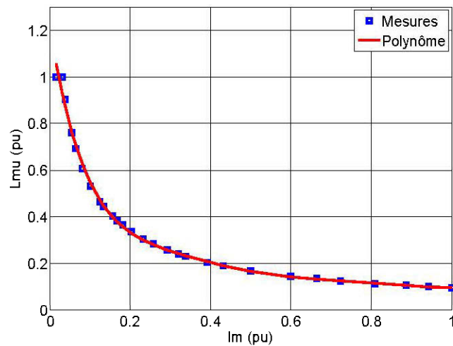
Figure 4-6 : Évolution de l'inductance de magnétisation en fonction de courant de magnétisation.
