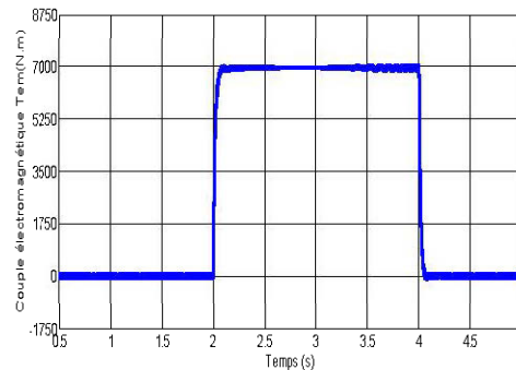
Figure 5-8 : Couple électromagnétique produit par la génératrice
