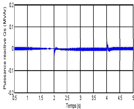
Figure 5-7 : Puissance réactive statorique
