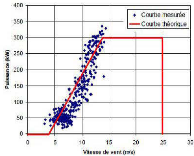
Figure 2-11 : Caractéristique de réglage d'une éolienne à vitesse fixe de 300 kW
