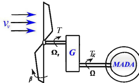
Figure 3-2 : Schéma de la turbine éolienne
