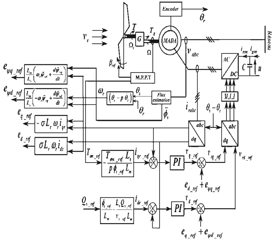
Figure 6-4 : Le schéma bloc du contrôle vectoriel modifié de la MADA
